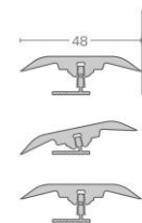
vyrovnávací profil pro Modular ONE
